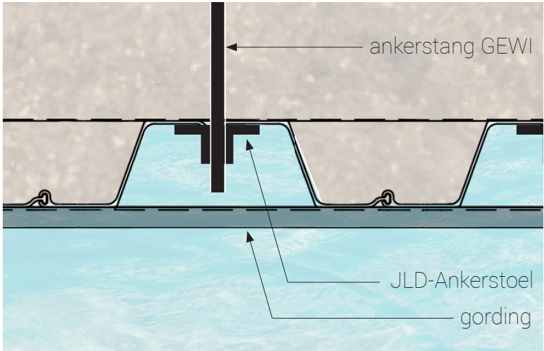
DETAIL BOVENAANZICHT
