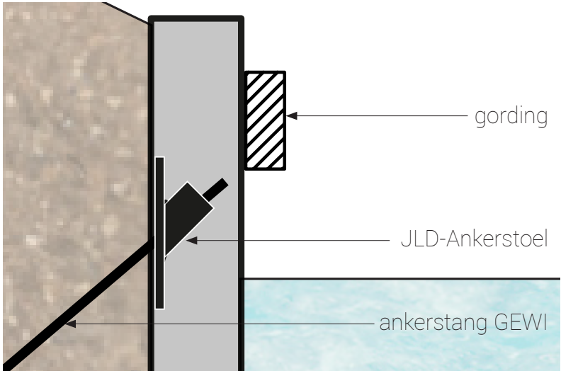
DETAIL ZIJAANZICHT
