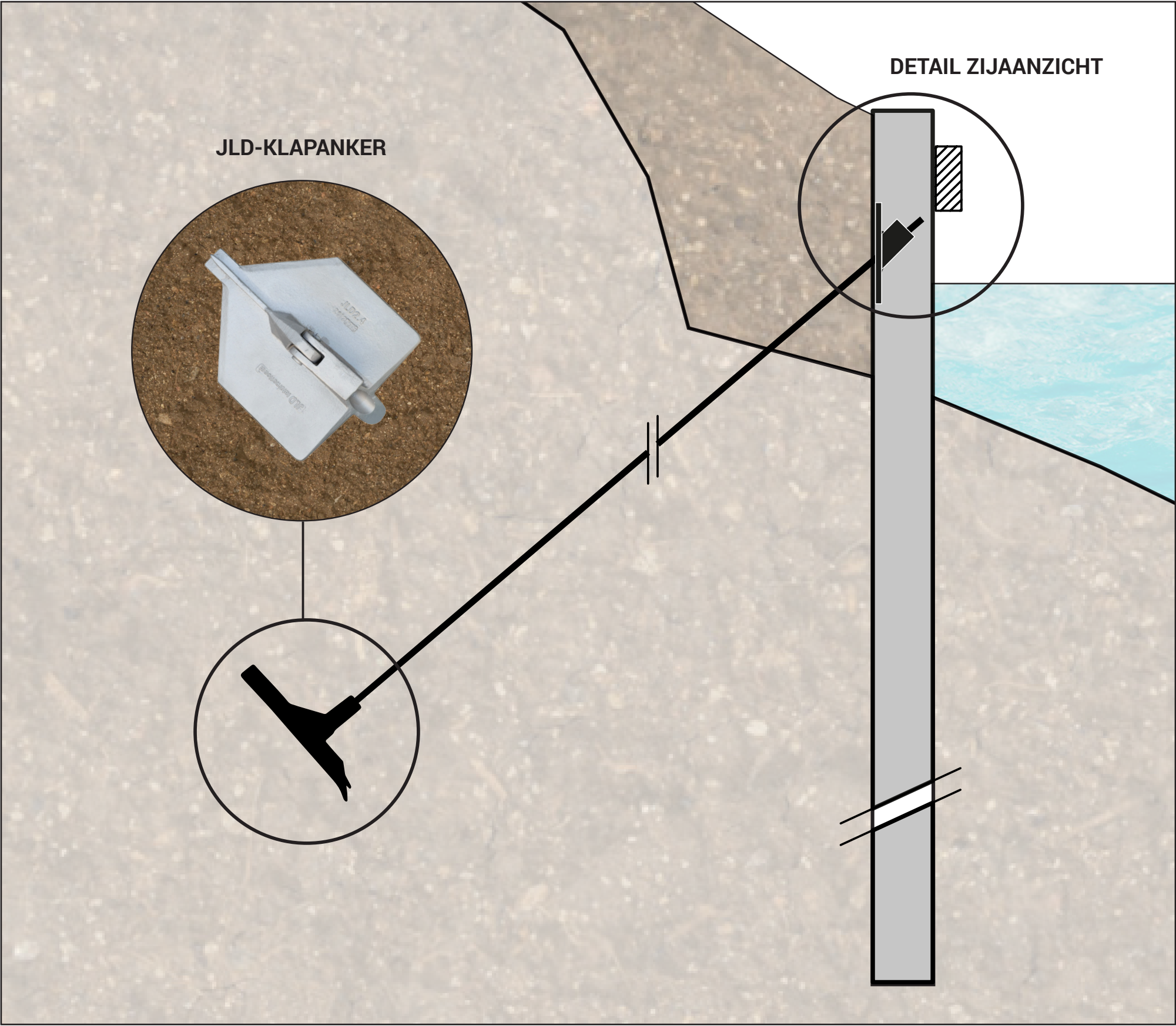
DETAIL VERANKERING DAMWAND : JLD-ANKERSTOEL
