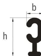
Hoekstuk C00
