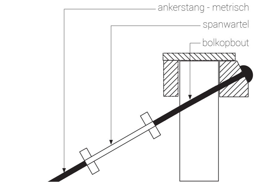
DETAIL ZIJAANZICHT
