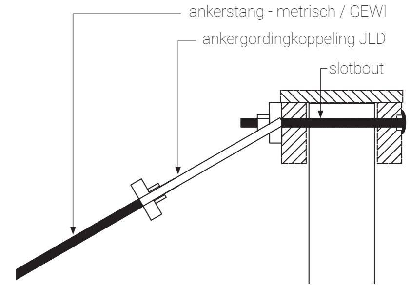
DETAIL ZIJAANZICHT
